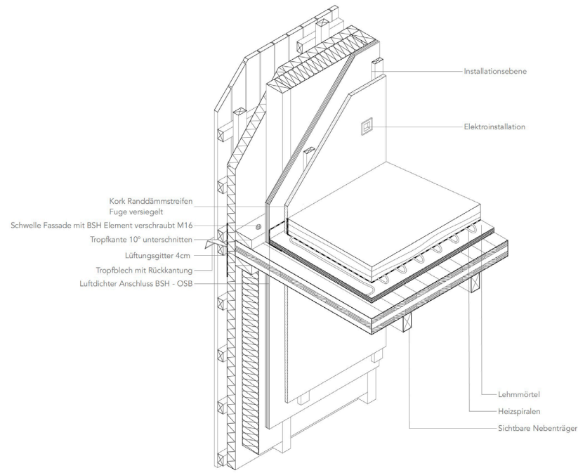
D.05 Anschluss Wand - Decke
