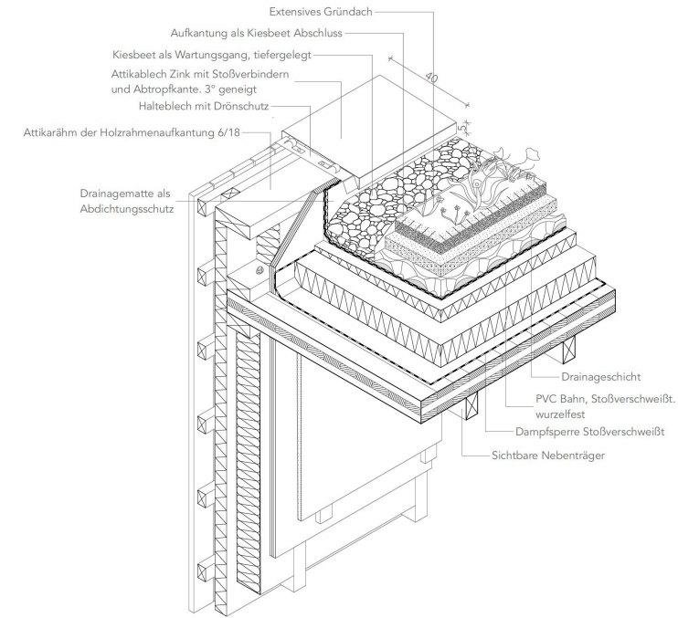
D.06 Anschluss Wand - Dach
