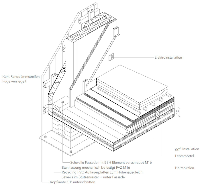
D.04 Anschluss Wand - Sohle
