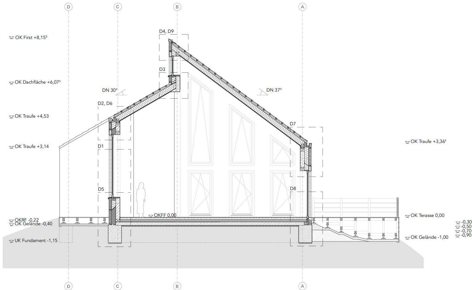
Schnitt A-A
