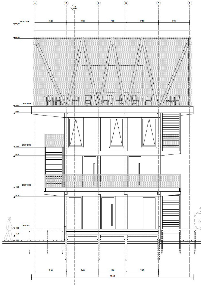
Ansicht Süd M 1:100
