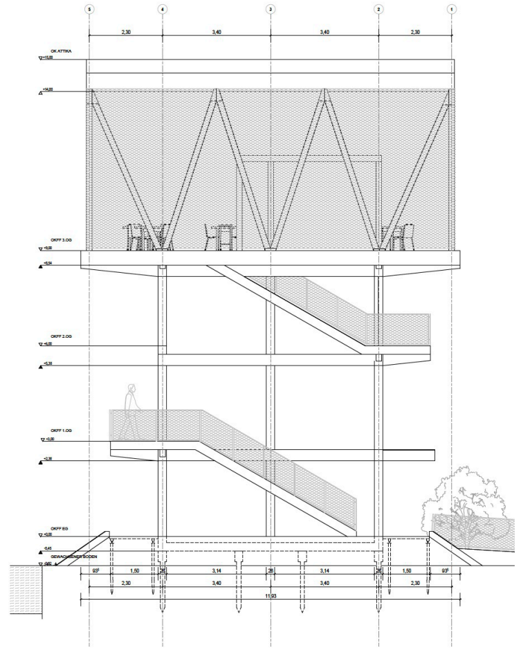
Ansicht Ost M 1:100
