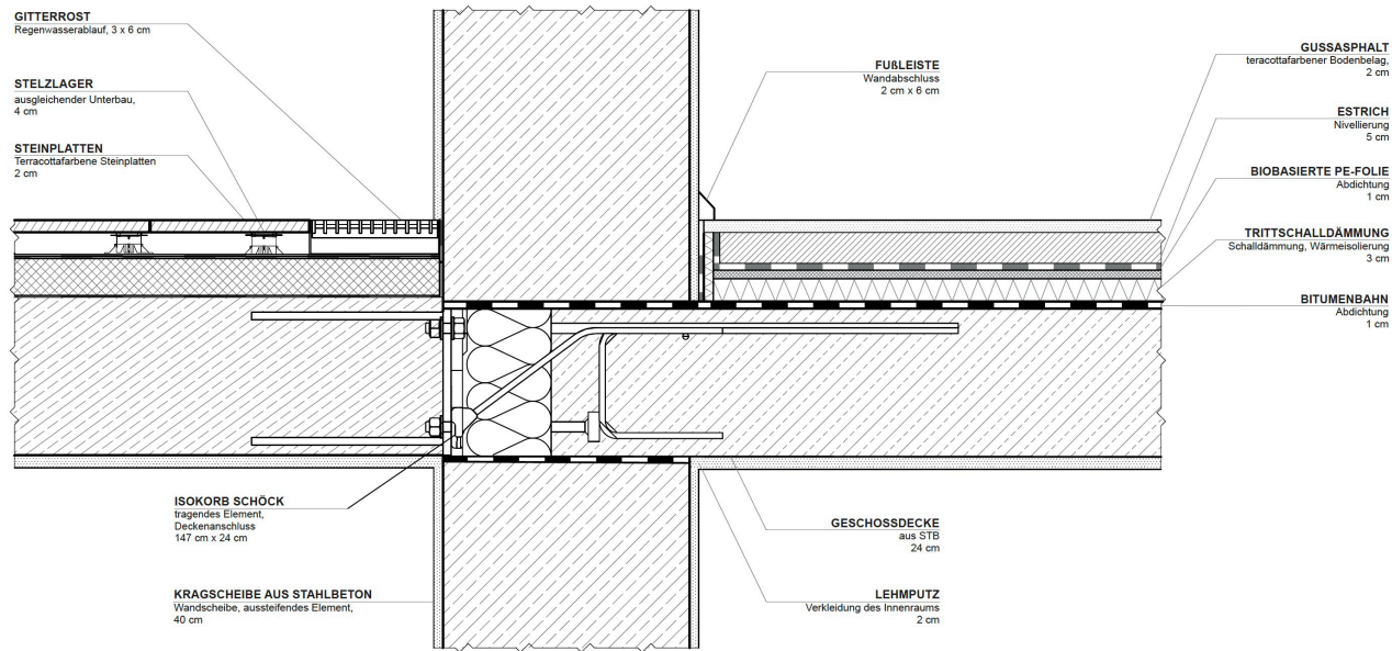
D-006 KRAGSCHEIBE VERTIKAL (M 1:5)
