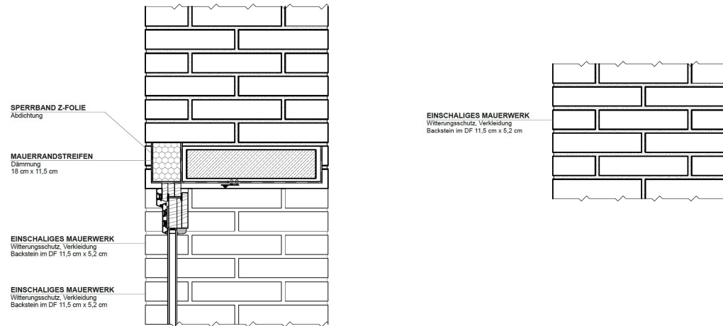
WANDAUFBAU EINSCHALIGES MAUERWERK (M 1:5)
