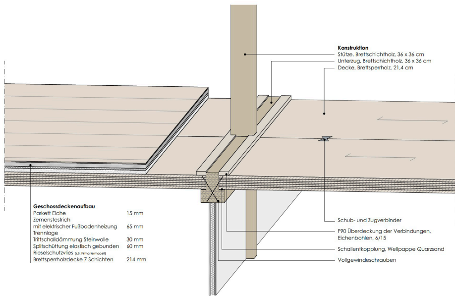
ISOMETRIE HOLZVERBINDUNG
