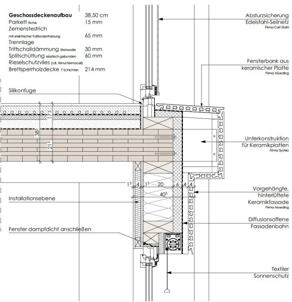
DETAIL KERAMIKFASSEDE | M 1:10
