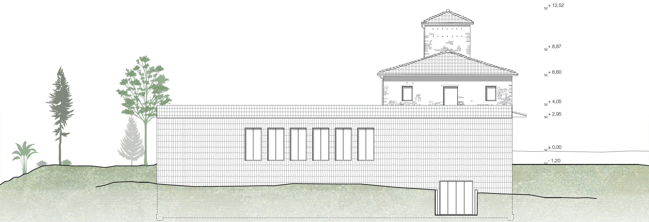
Ansicht 02 | Nord-West | M 1:100
