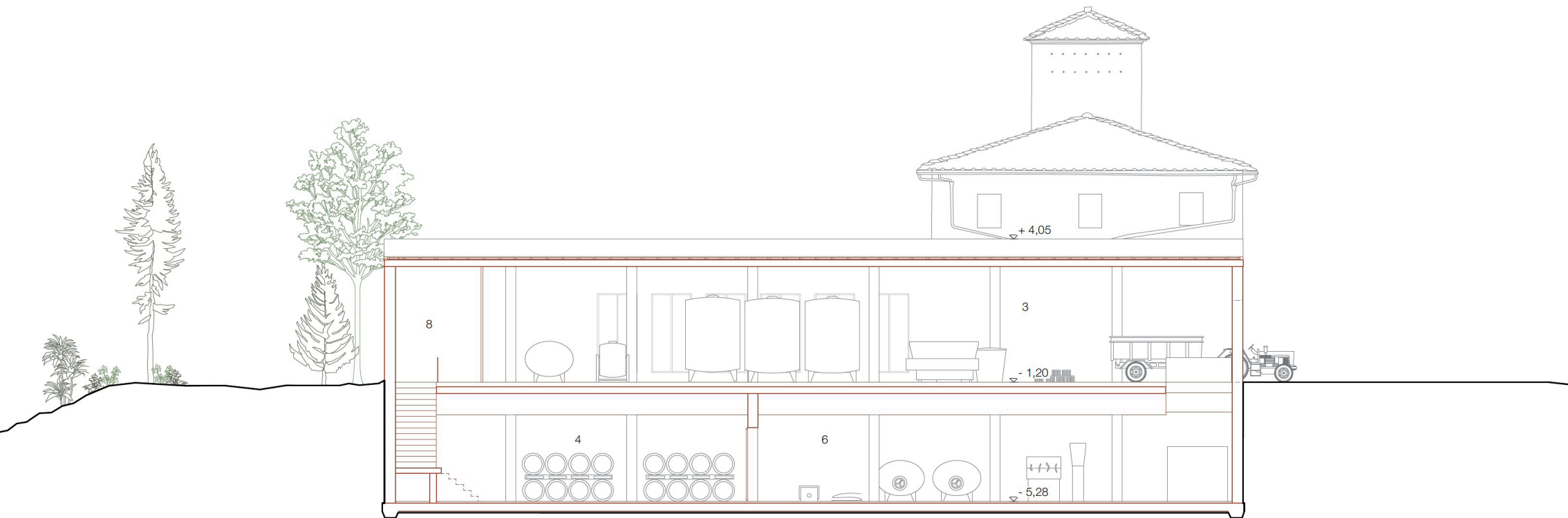
Schnitt C-C | Weinproduktion | M 1:100
