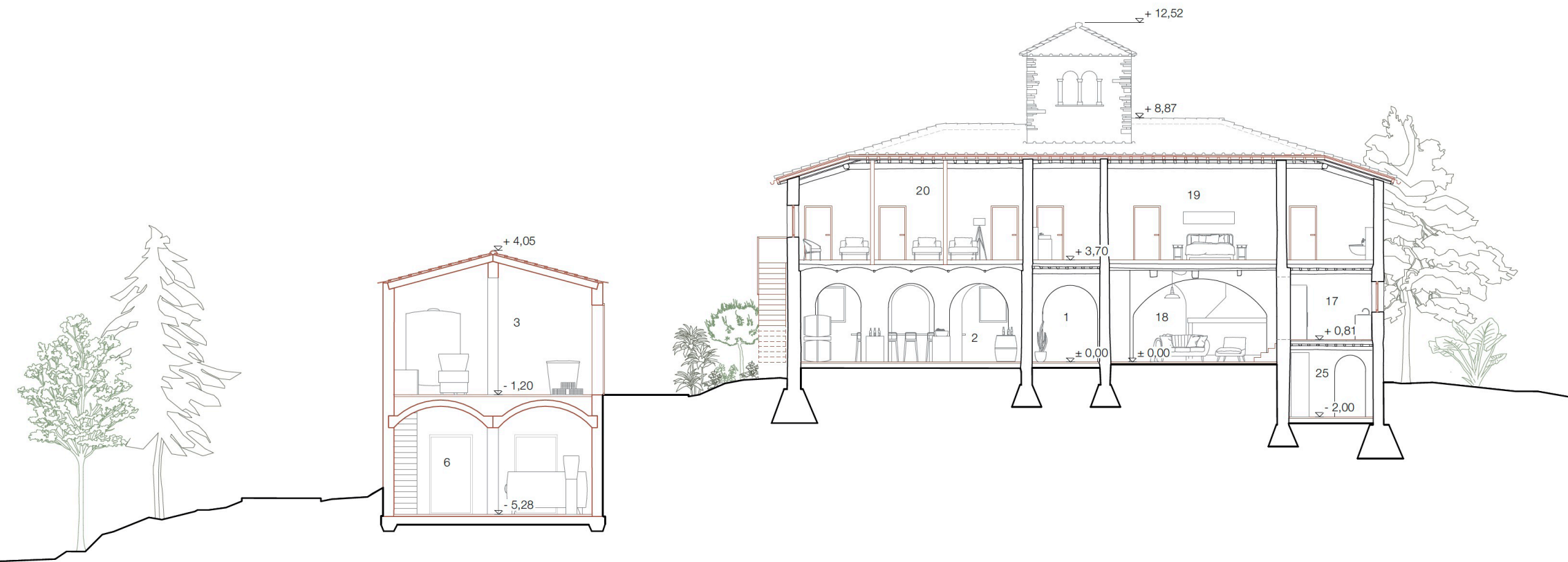
Schnitt A-A | Weinproduktion - Haupthaus | M 1:100
