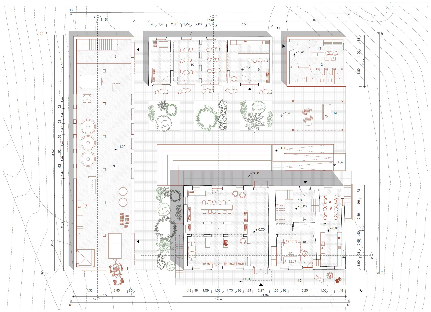
Grundriss Erdgeschoss | M 1:100
