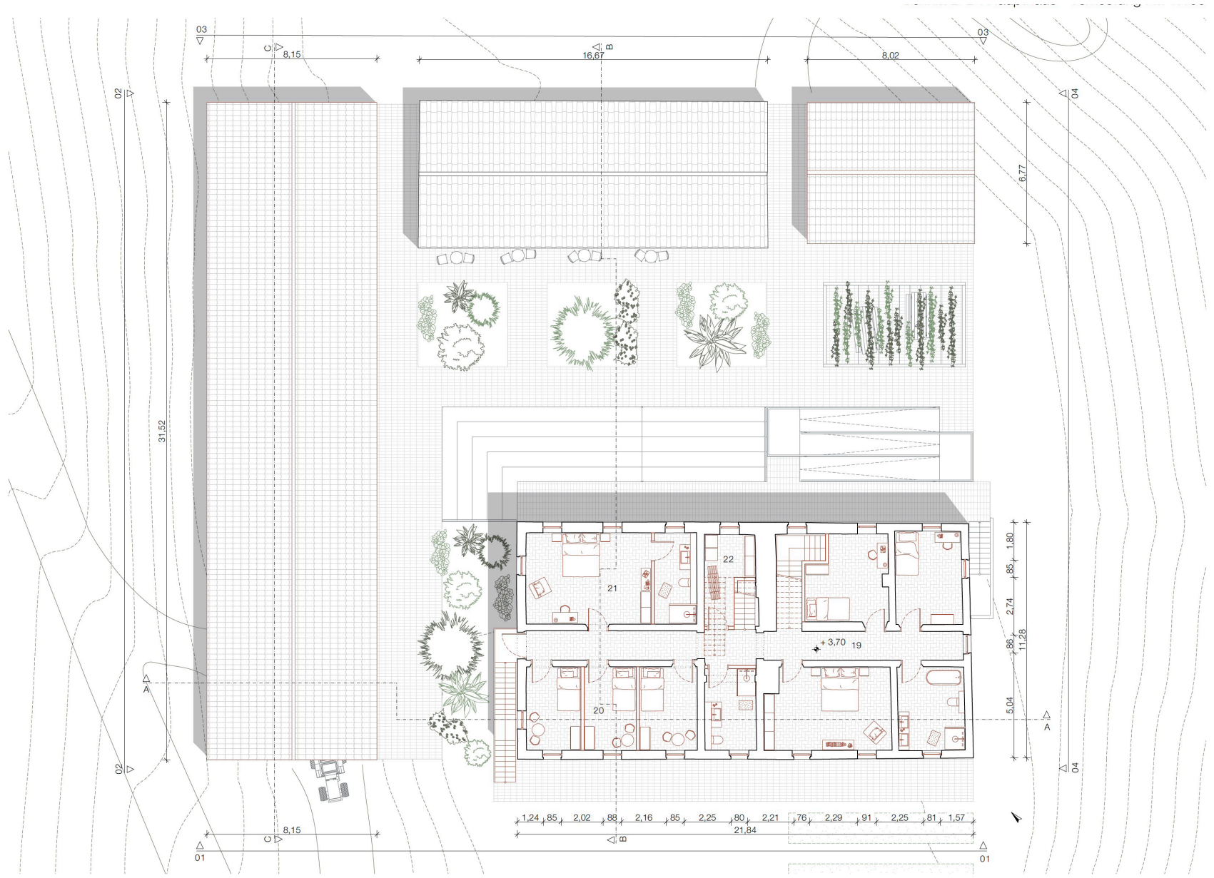
Grundriss Obergeschoss I M 1:100
